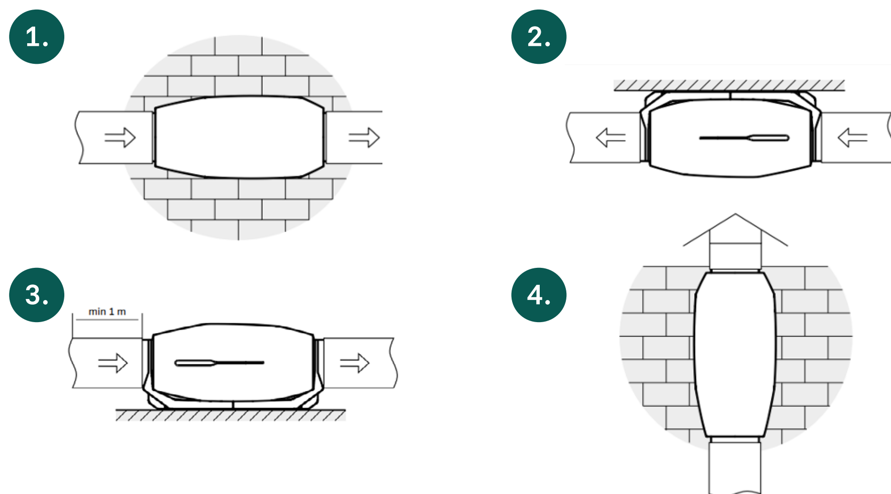
1. Montaż ścienny poziomy | 2. Montaż sufitowy | 3. Montaż na podłodze | 4. Montaż ścienny pionowy
