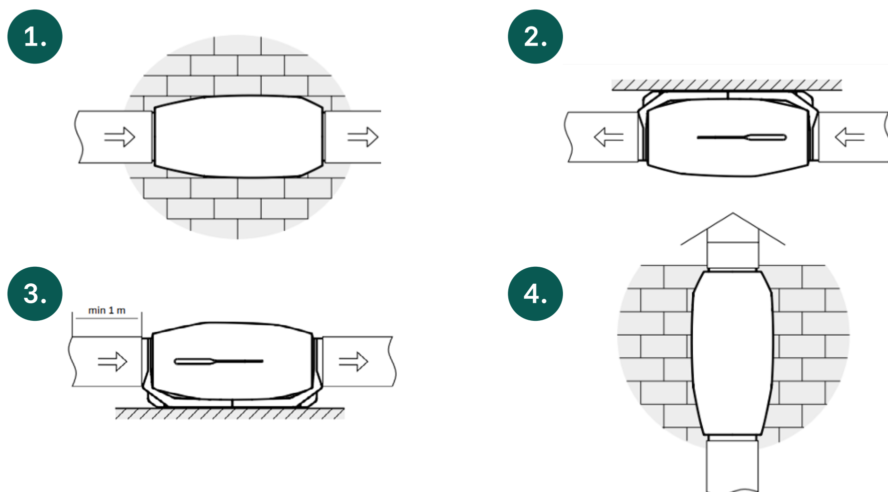
1. Horizontale Wandmontage | 2. Deckenmontage | 3. Montage auf dem Boden | 4. Vertikale Wandmontage
